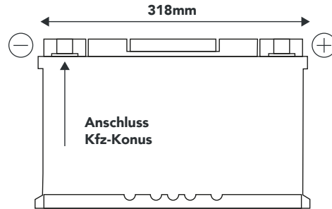
Abmaße: Länge 318mm | Breite 175mm | Höhe 190mm
